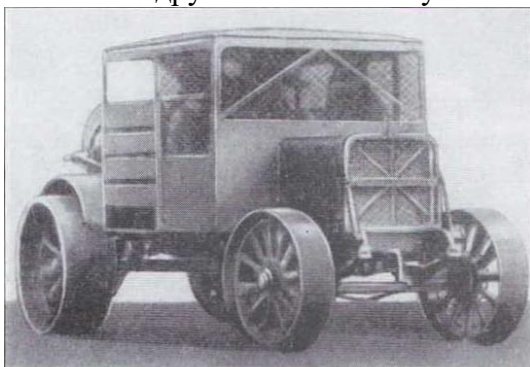
«Руссо-Балт Т 40/60» — первый артиллерийский тягач отечественного производства с бензиновым двигателем мощностью 60 л.с. 1913 г.
