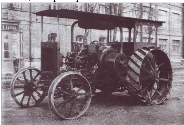
Колесный трактор с керосиновым двигателем производства Коломенского машиностроительного завода. 1917 г.
