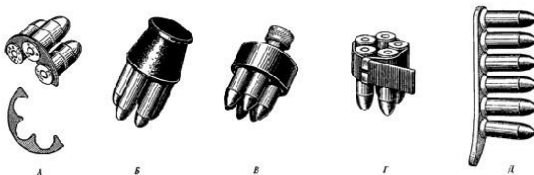
Ускорители заряжания револьверов: А — металлические обоймы для патронов, не имеющих фланцев; Б — резиновый усечённый конус, освобождающий введенные в камеры патроны после нажима на верхнее основание; В — ускоритель, в котором патроны удерживаются и освобождаются с помощью вращающейся головки; Г — лента, отделяемая от патронов после введения их головных частей в камеры; Д — плоская эластичная обойма, служащая для
