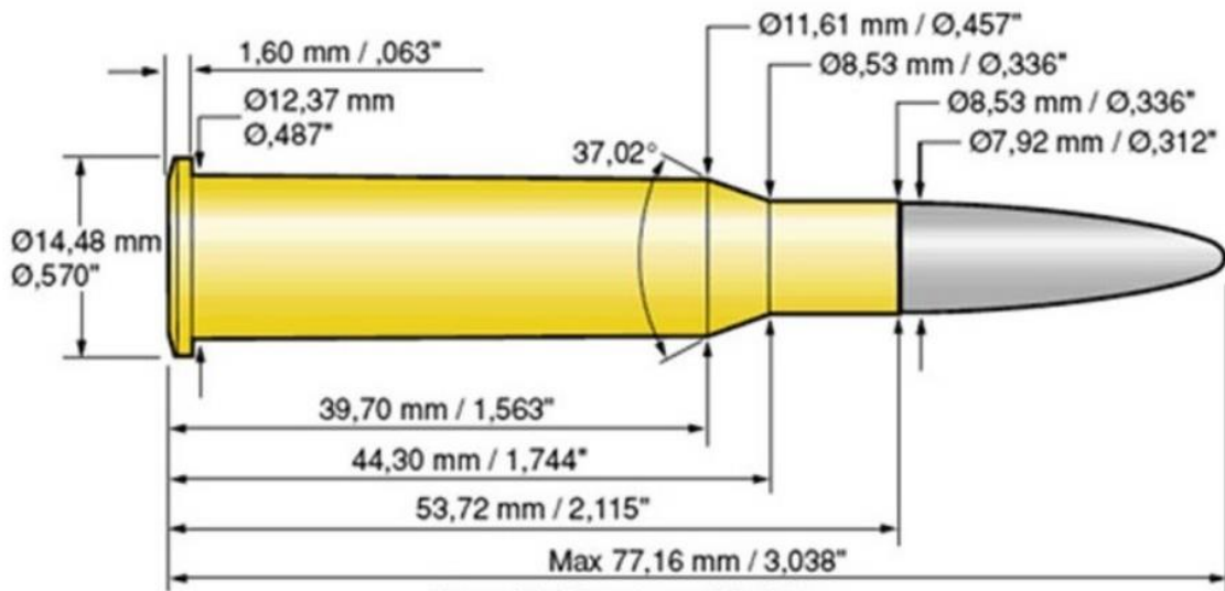
Рисунок 2.1 – Схема патрона 7,62 × 54 мм
