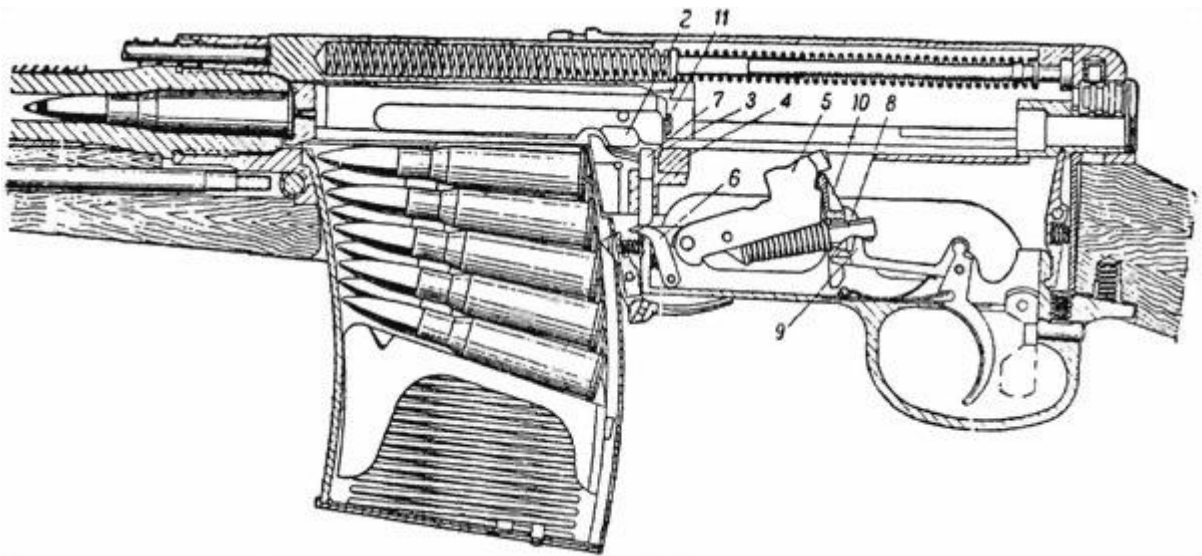
Система самозарядной винтовки Токарева СВТ-38/40 АВТ-40
