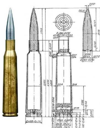
Патрон В.Г. Федорова калибра 6,5×57 мм
