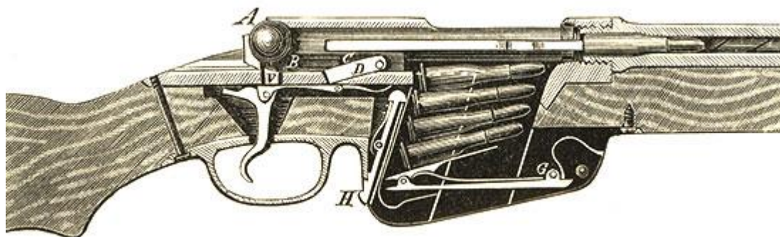
Система Манлихера образца 1886 года (M1886 калибра 11x58 мм R и M1886-90 калибра 8x52 R)
