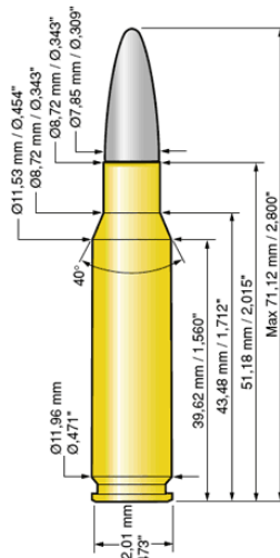
Патрон 7,62x51 мм / .308 Winchester, 1947, США
