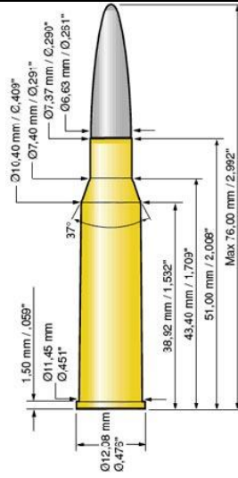
Патрон 6,5×51 мм Арисака
