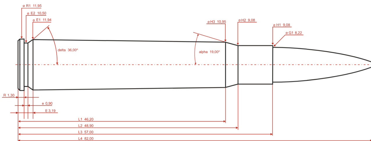
7,92x57 мм Маузер. Все размеры в миллиметрах.
