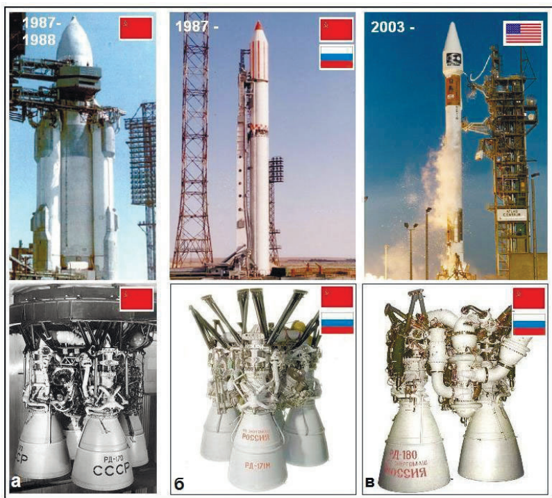
Лунное наследство СССР – 3. Двигатели от «Энергии» на других ракетах. а) советская ракета «Энергия» и её двигатель, б) советская (российская) ракета «Зенит» и её двигатель, в) г) американская ракета «Атлас» с российским двигателем РД180
