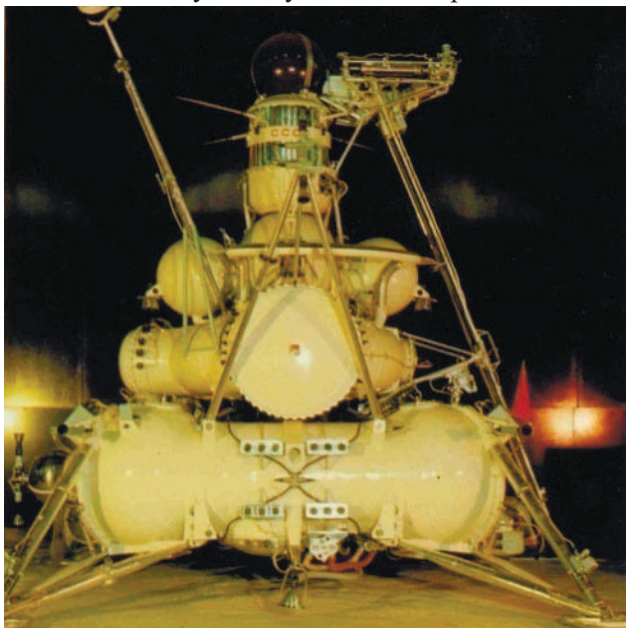
АМС Е-8-5 для доставки лунного грунта («Луна-15 и др.) («К звёздам», «Планета», Москва, 1980, с.98)
